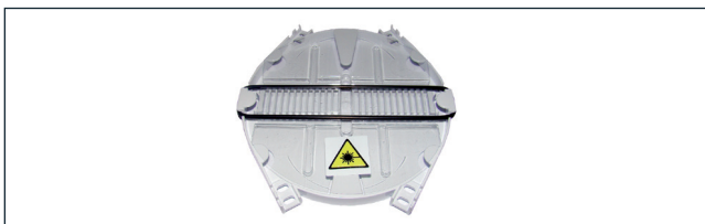
Cassette de empalme para 12/24 fusiones (Ref. 5190)
